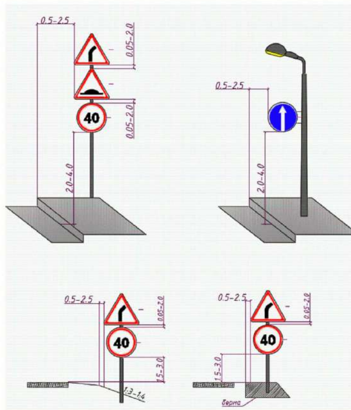
Рисунок 3 – Способы установки дорожных знаков
