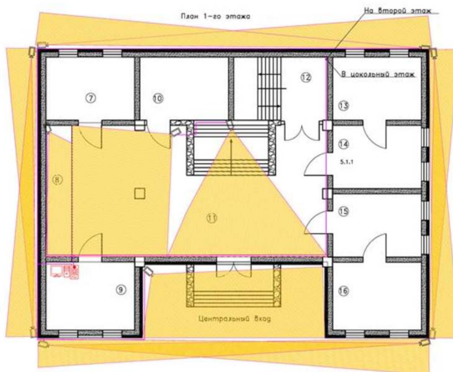
План расположения видеокамер СОТ в помещении
